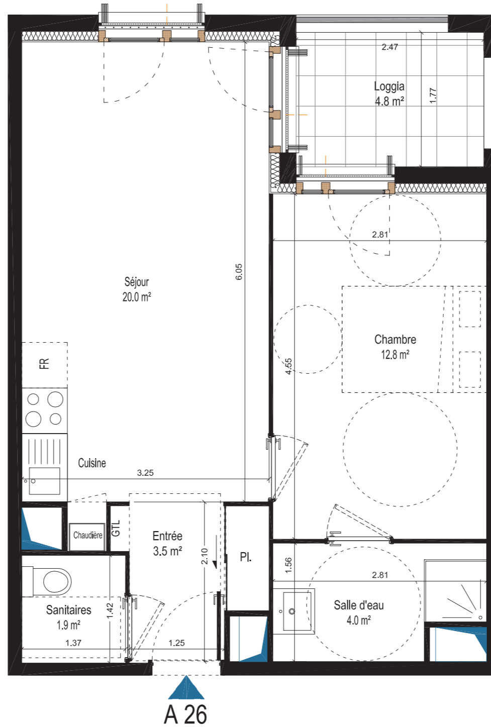
Plan du 2ème étage
